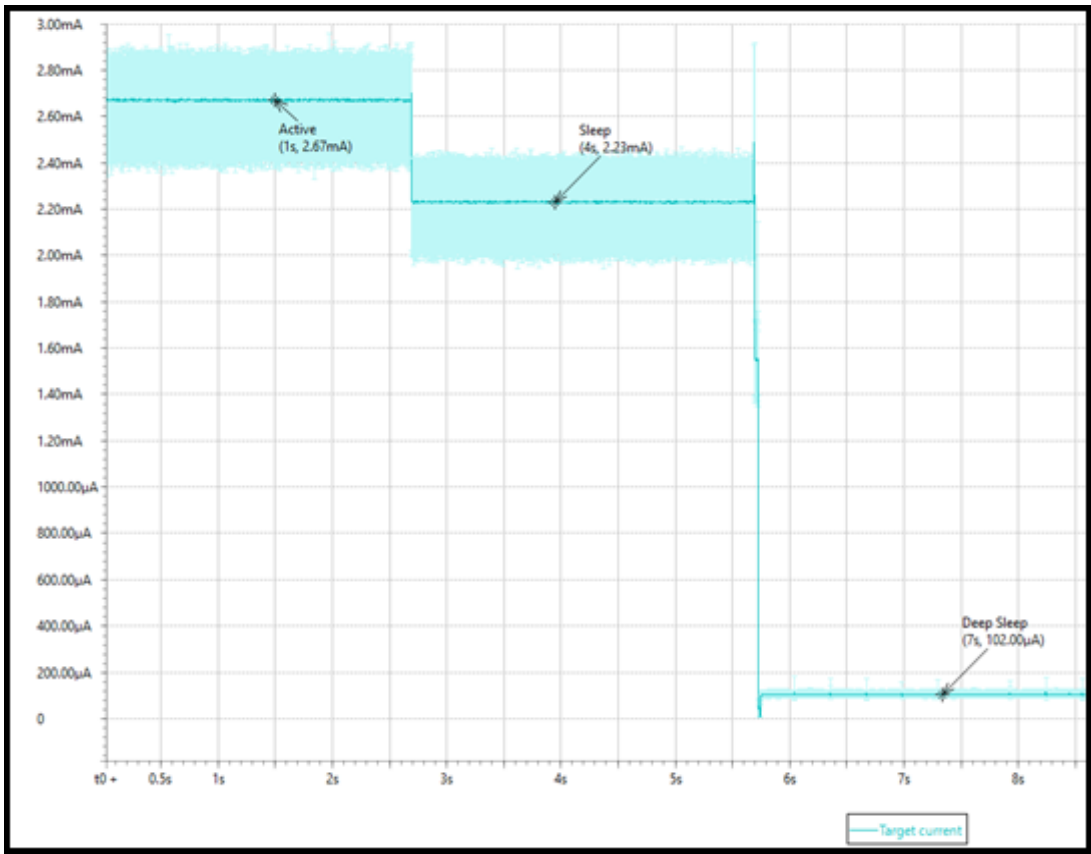
图12. MCU-Link的能耗测量窗口
